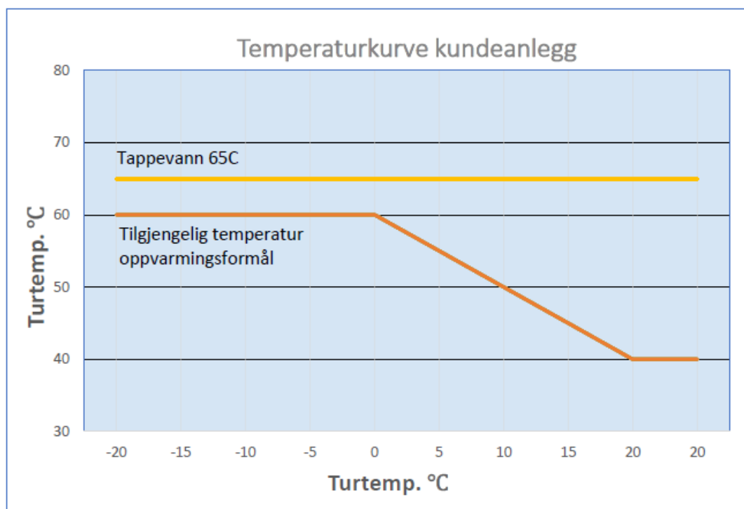
Figur 2: Eksempel på utetemperaturkompensert varmekurve for kundenanlegg.
